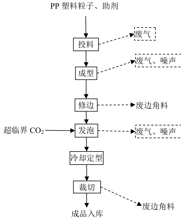
图2-2 项目生产工艺流程图
